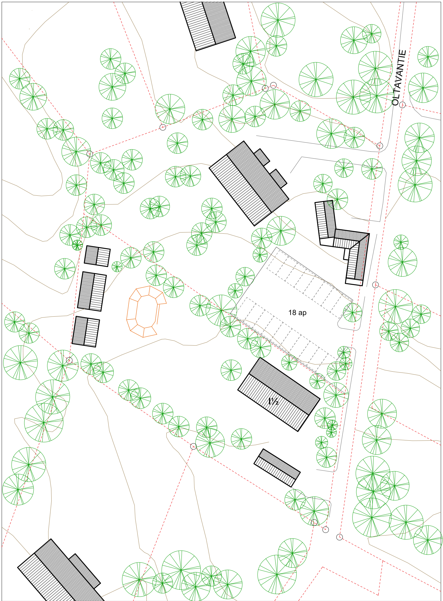
Oltavantie 4 HAVAINNEKUVA, versio B 1/500 Valtteri Heinonen, 8.2.2021
